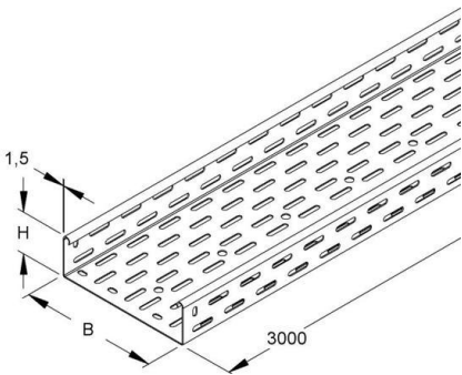
Maßzeichnung
