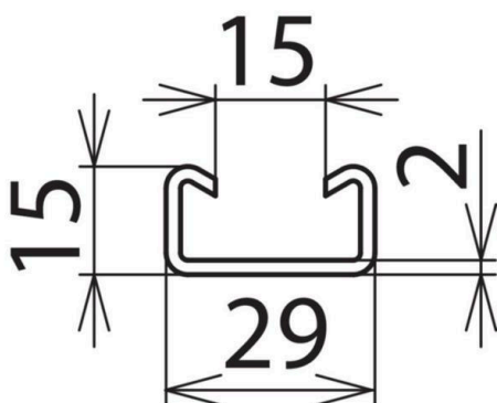
Maßzeichnung
