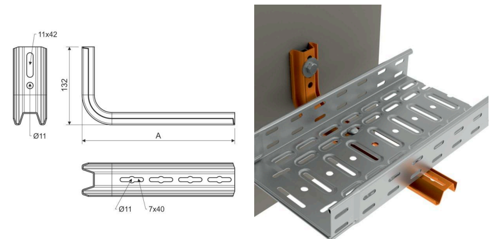
Maßzeichnung
