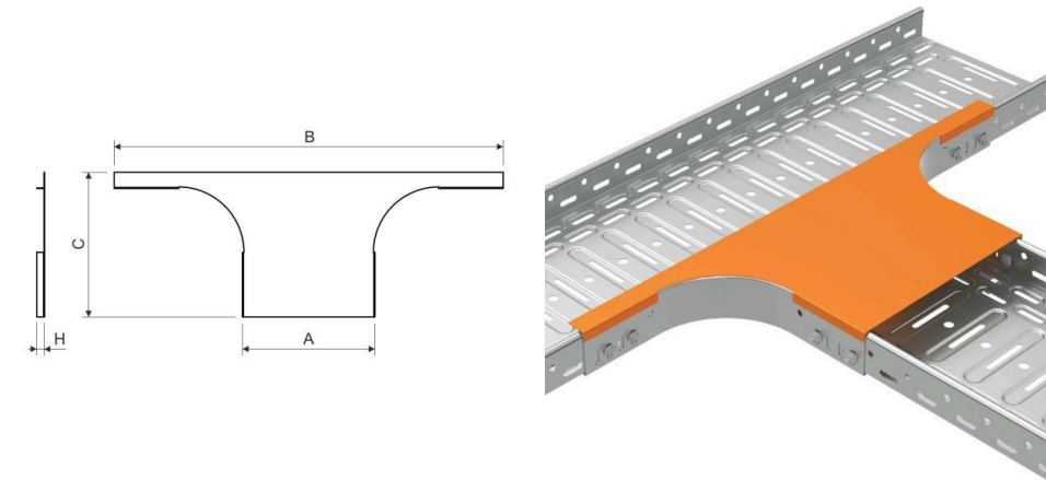
Maßzeichnung
