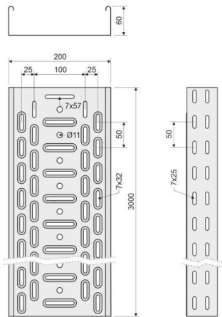
Maßzeichnung
