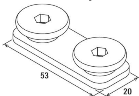
Maßzeichnung
