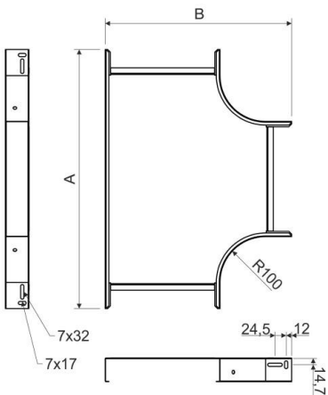
Maßzeichnung
