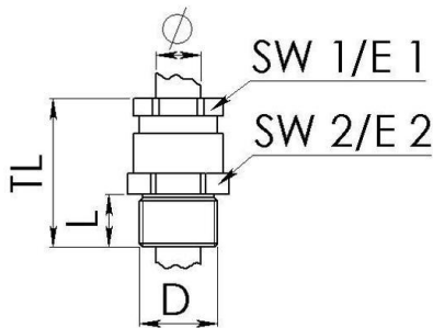
Maßzeichnung
