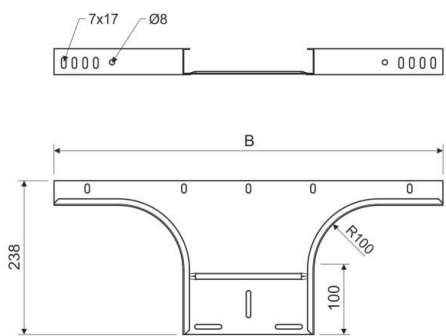
Maßzeichnung
