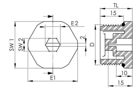
Maßzeichnung
