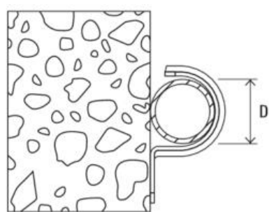
Strichzeichnung
