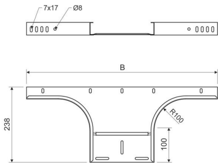
Maßzeichnung
