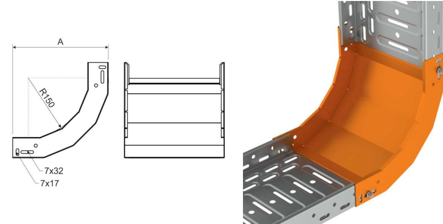
Maßzeichnung
