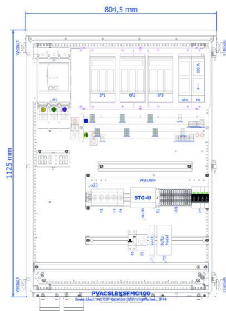
Maßzeichnung
