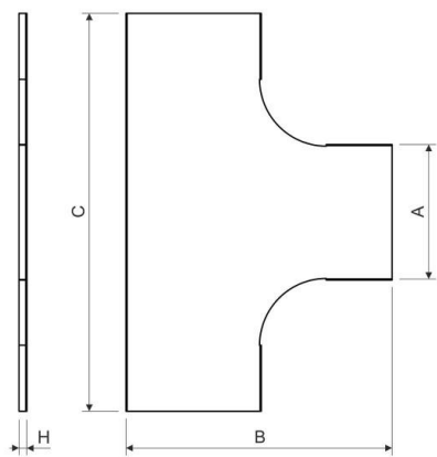
Maßzeichnung
