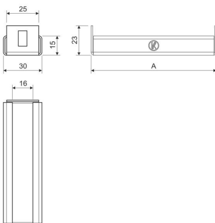
Maßzeichnung
