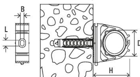
Strichzeichnung
