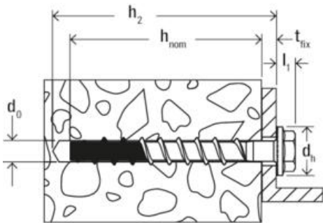
Strichzeichnung
