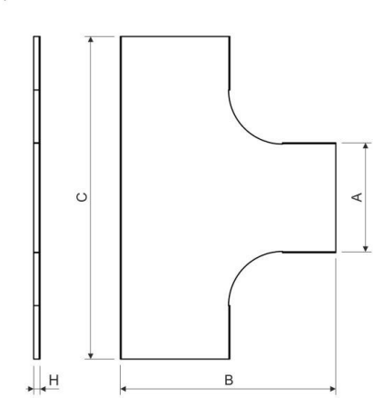
Maßzeichnung
