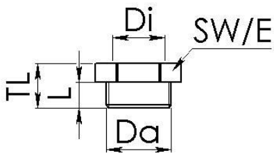
Maßzeichnung
