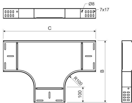
Maßzeichnung
