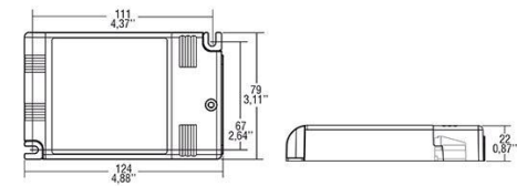
Maßzeichnung
