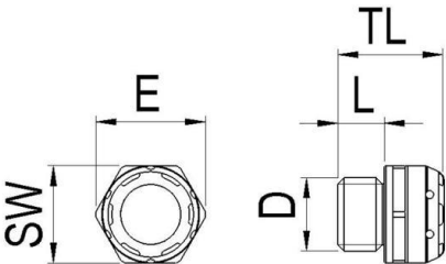
Maßzeichnung
