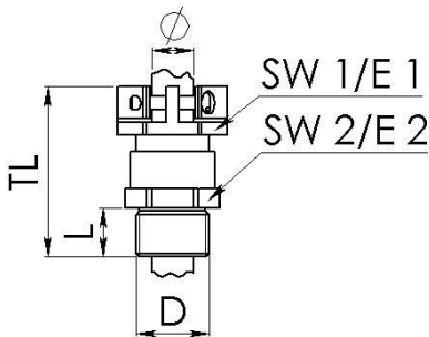
Maßzeichnung
