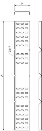
Maßzeichnung
