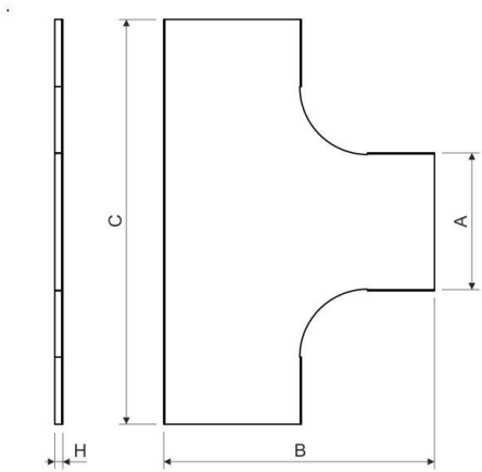
Maßzeichnung
