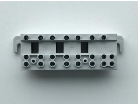
Zaehlersteckleiste Wienstrom ZSK-GS80
