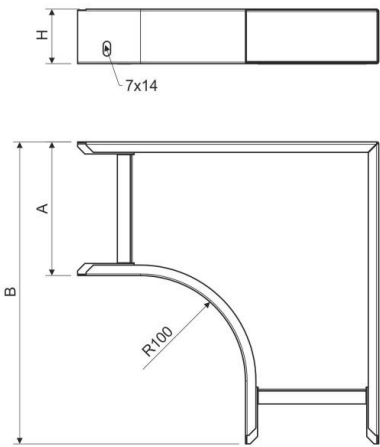
Maßzeichnung
