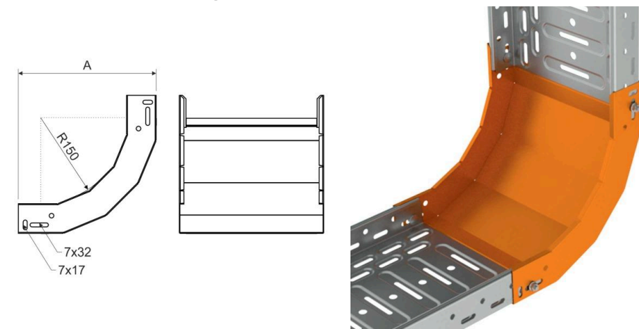
Maßzeichnung
