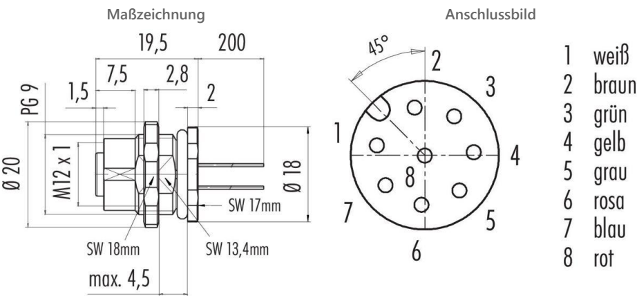
Ausführung mit Zink Druckgussgehäuse
