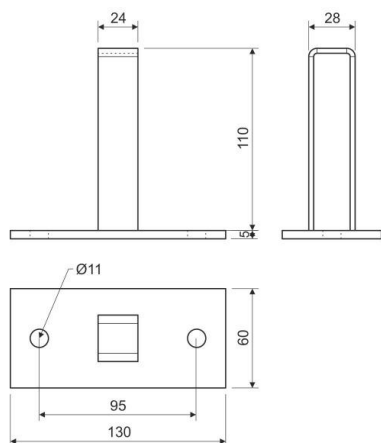
Maßzeichnung
