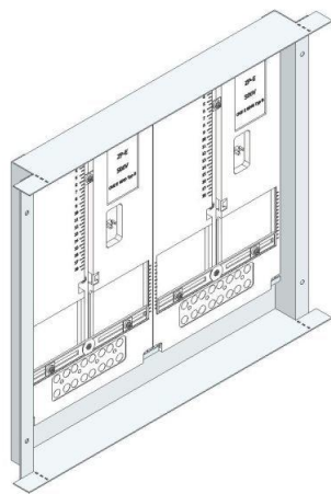
Zählerwanne mit Zählerplatte
