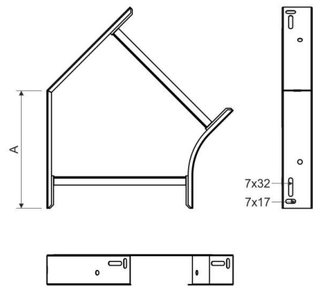
Maßzeichnung
