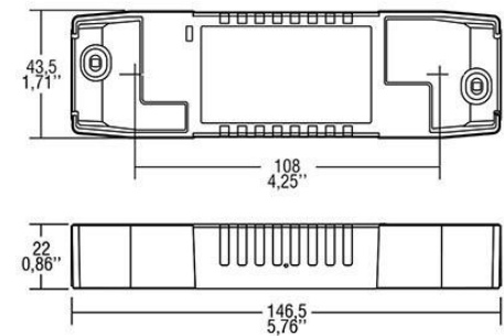
Maßzeichnung
