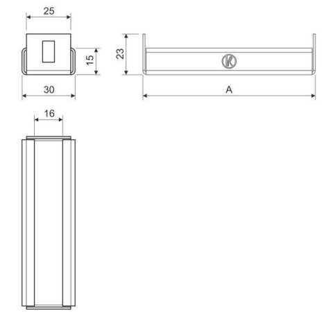
Maßzeichnung
