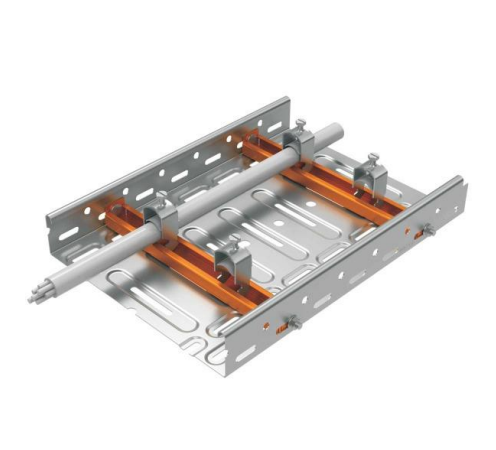
Produktbild Detailsicht
