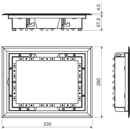
Maßzeichnung
