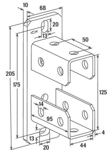
Maßzeichnung
