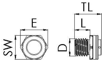
Maßzeichnung
