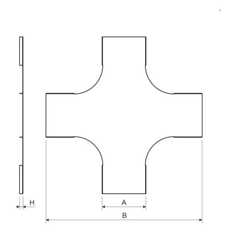
Maßzeichnung
