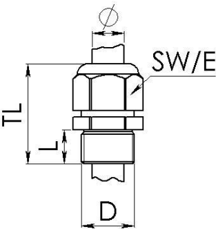
Maßzeichnung
