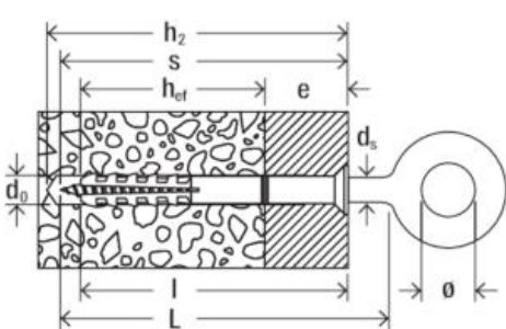
Strichzeichnung
