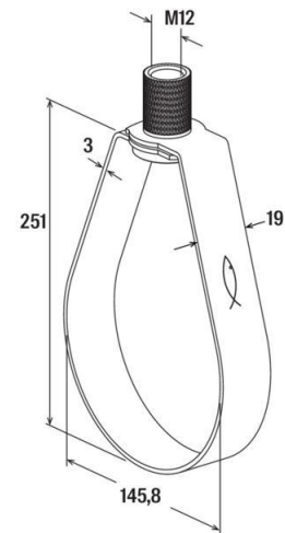
Maßzeichnung
