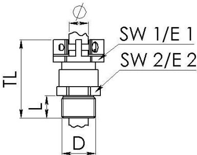
Maßzeichnung
