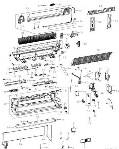
Explosionszeichnung
