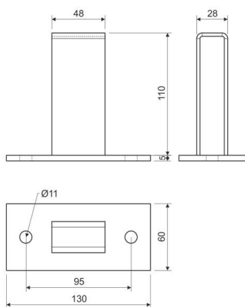
Maßzeichnung
