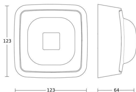
Maßzeichnung
