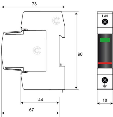
Maßzeichnung
