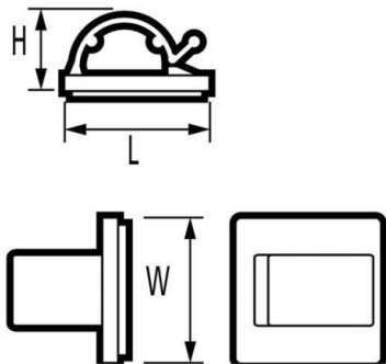
Maßzeichnung
