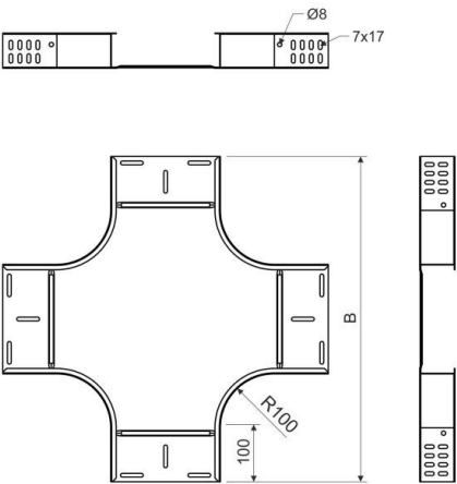
Maßzeichnung
