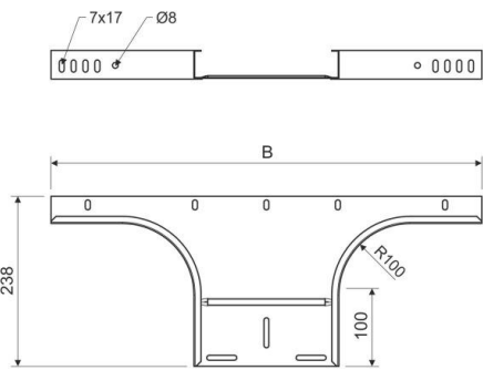
Maßzeichnung
